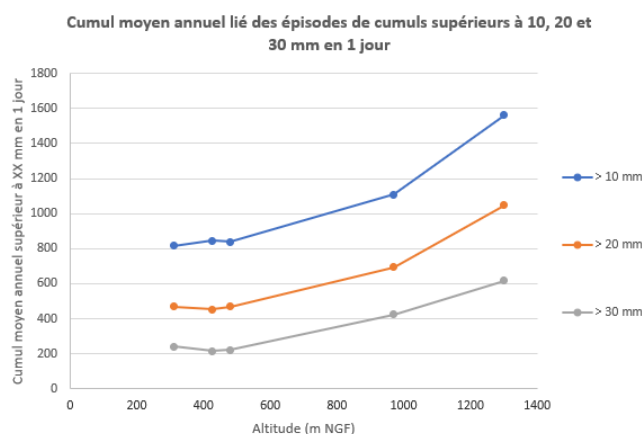
Evolution du cumul moyen annuel de pluie en fonction de l'altitude
