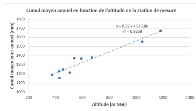
Evolution du cumul moyen annuel de pluie en fonction de l'altitude
